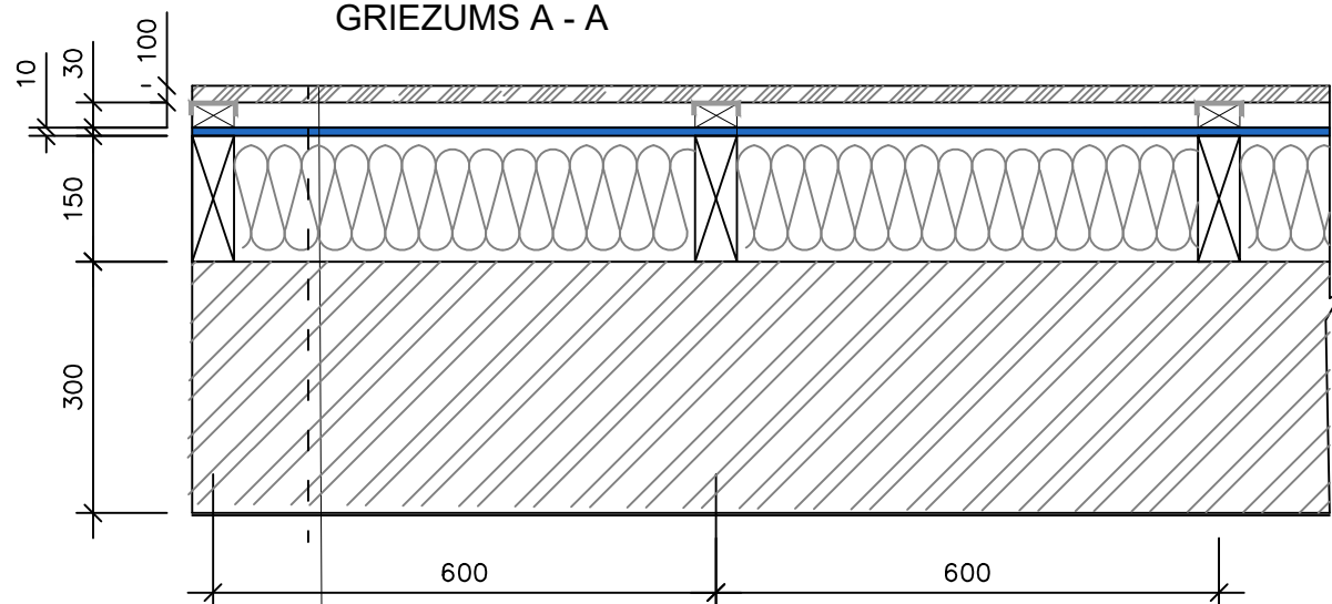
GRIEZUMS A - A
